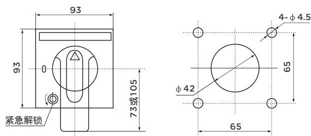
“F”型方形手柄外形柜门开孔尺寸(开孔中心离铰链距离不小于100mm)
