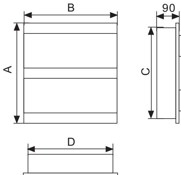
20、24、30、45回路暗装式
