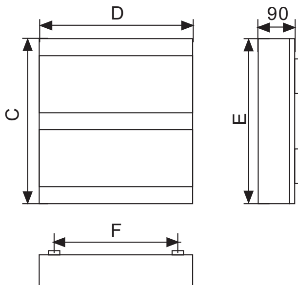
20、24、30、45回路明装式
