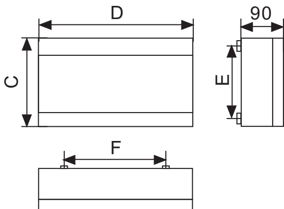
4、6、8、10、12、15、18回路明装式
