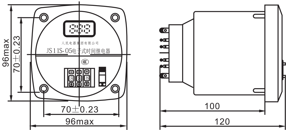
图3 JS11S-05(原JSS1P1-05/M)外形尺寸
