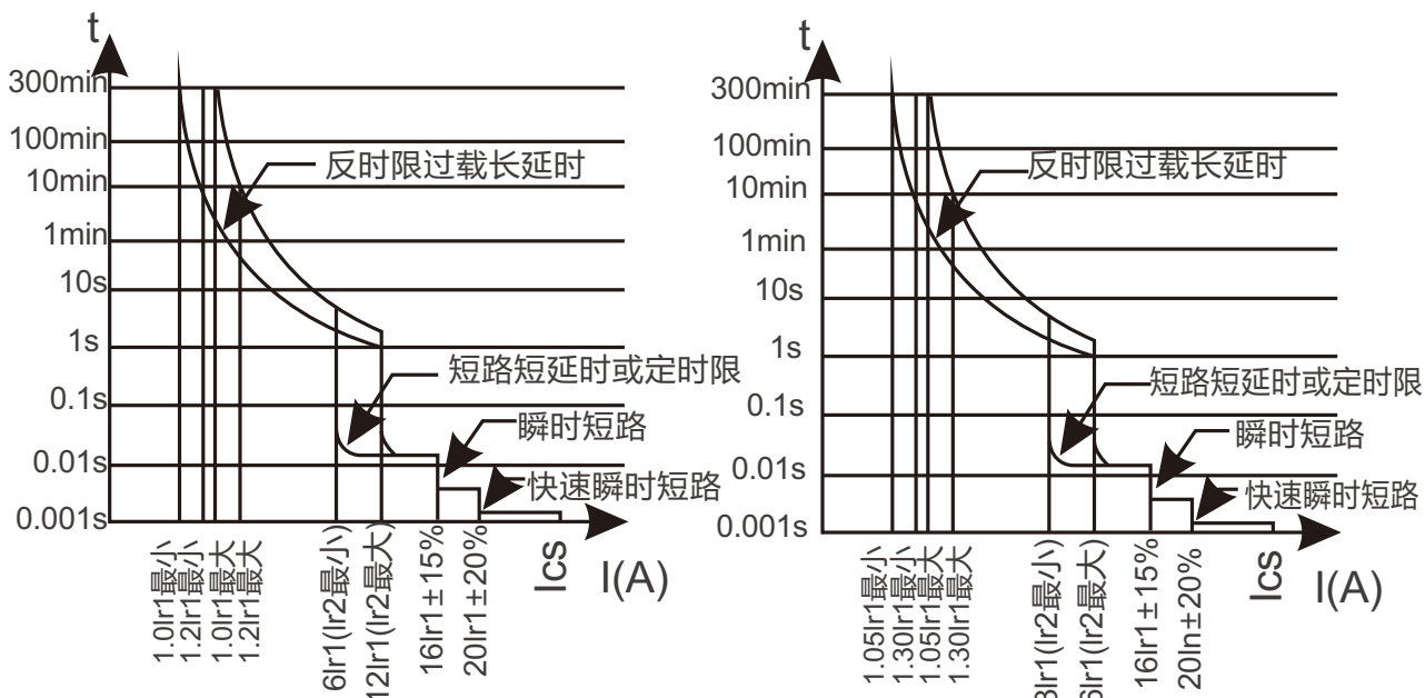
RDCPS电动机保护时间-电流特性
