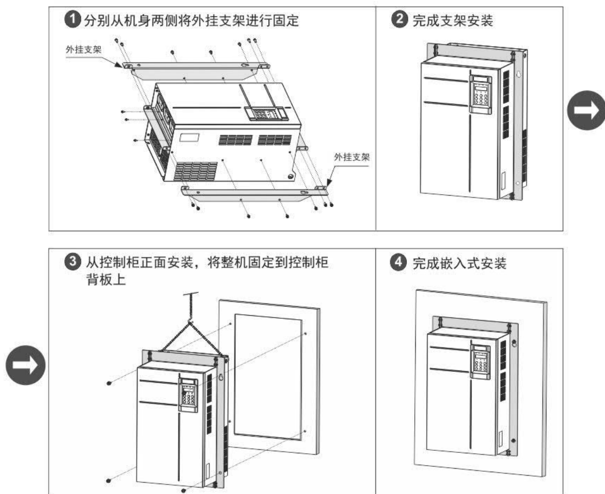
图 3-5 RDI67ST45G(B)~RDI67ST160G, RDI67S-2T22G(B)~RDI67S-2T55G 机型嵌入式安装示意图
