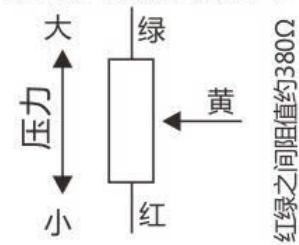
远传压力表等效图
