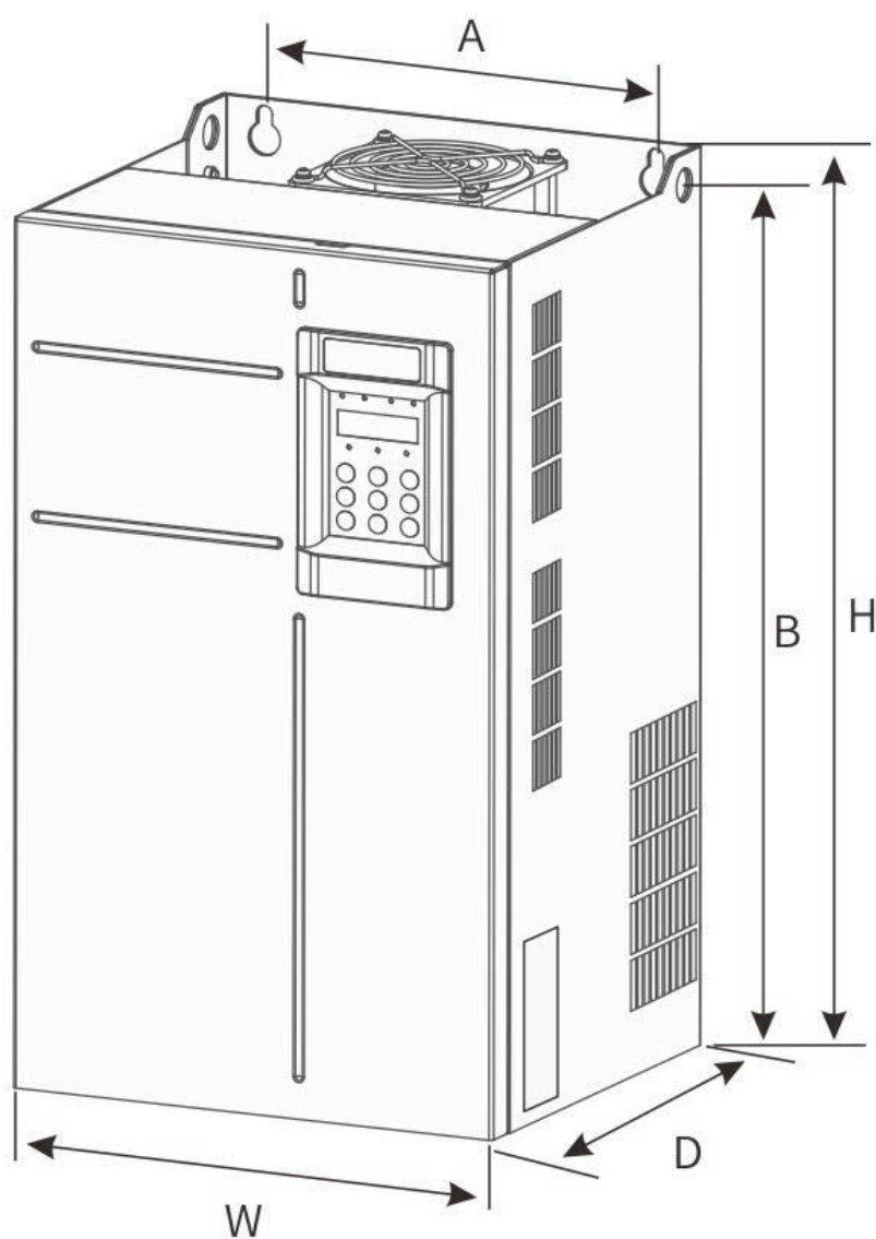
外形及安装尺寸示意图
