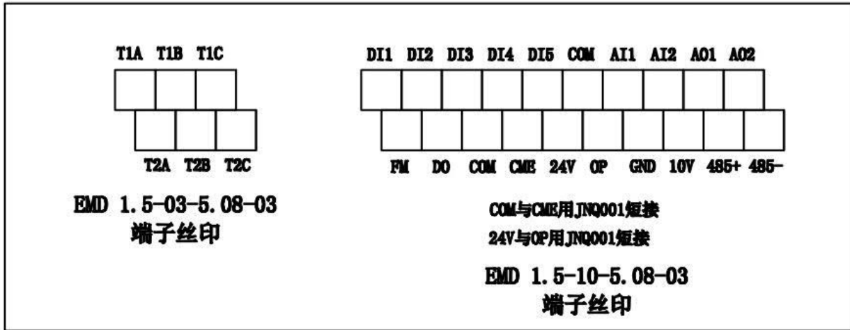
图3-10 15KW及以上控制端子图片
