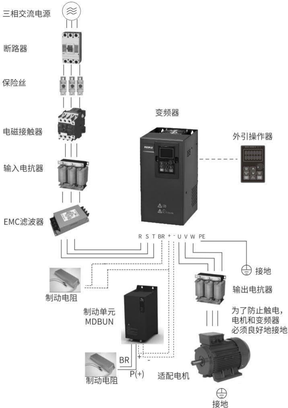
图 2-1 系列系统构成
