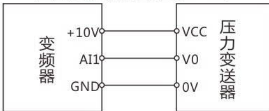
压力变送器接线图(0-5V)
