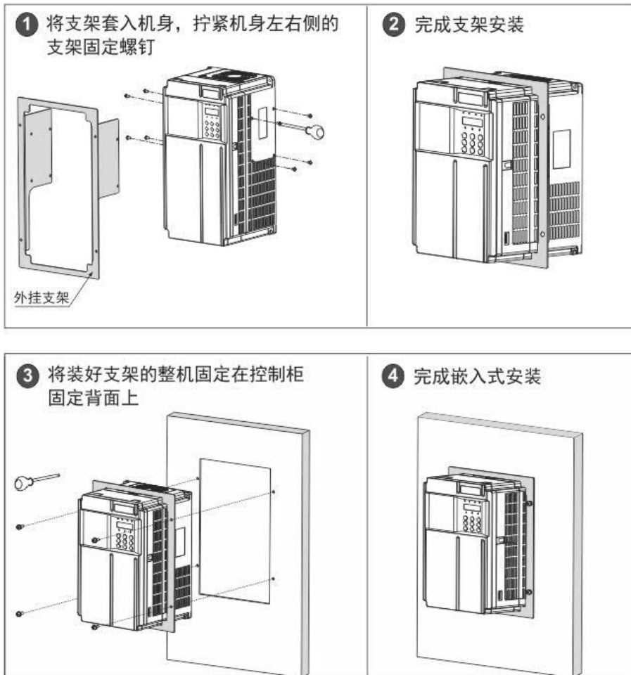
图 3-4 RDI67ST0.4GB~RDI67ST37G(B), RDI67S-2T0.4GB~RDI67S-2T18.5G(B)机型嵌入式安装示意图
