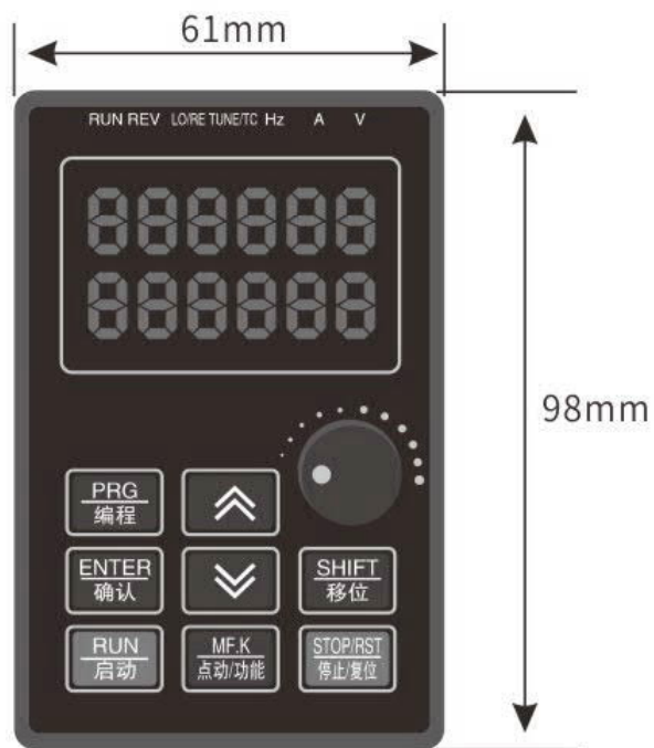
键盘开孔尺寸
