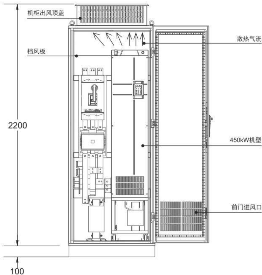
图 3-6 直排风机柜示意图
