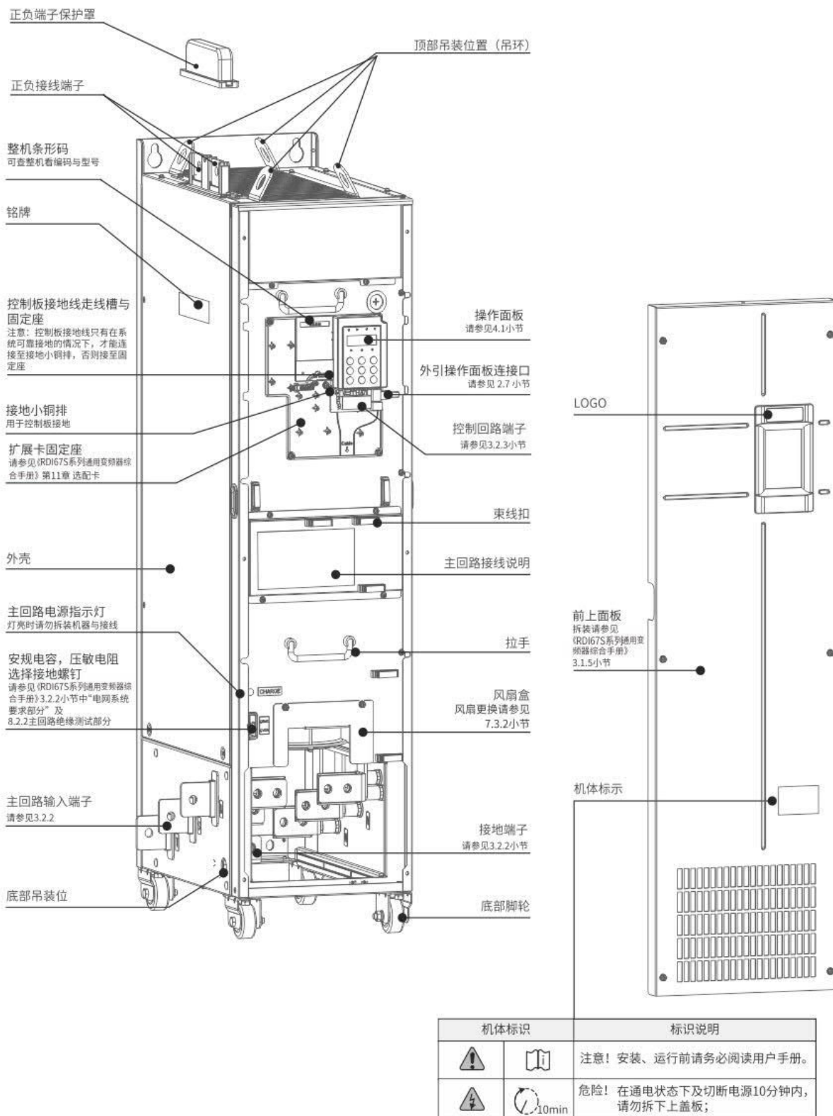
图 1-3 产品部件示意图【RDI67ST200G~RDI67ST450G】
