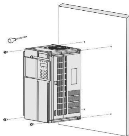
图 3-2 RDI67ST0.4GB~RDI67ST37G(B),RDI67S-2T0.4GB~RDI67S-2T18.5G(B) 机型壁挂式安装示意图
