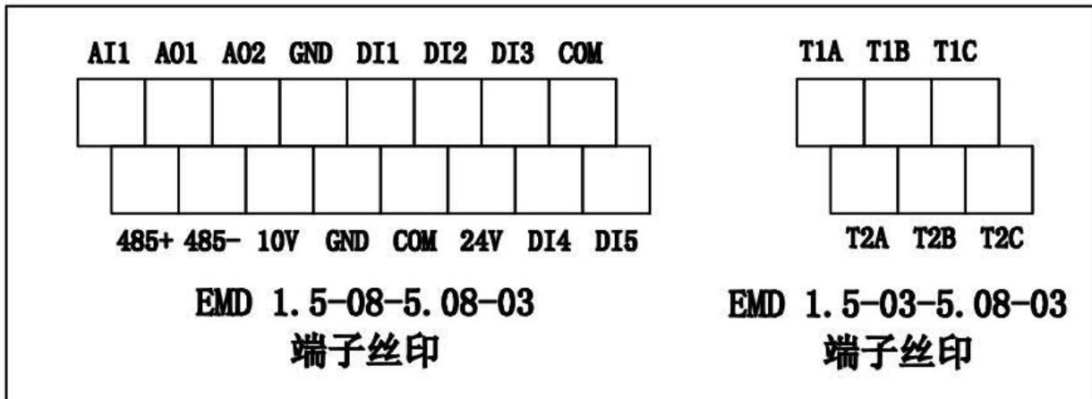
图3-11 11KW及以下控制端子图片
