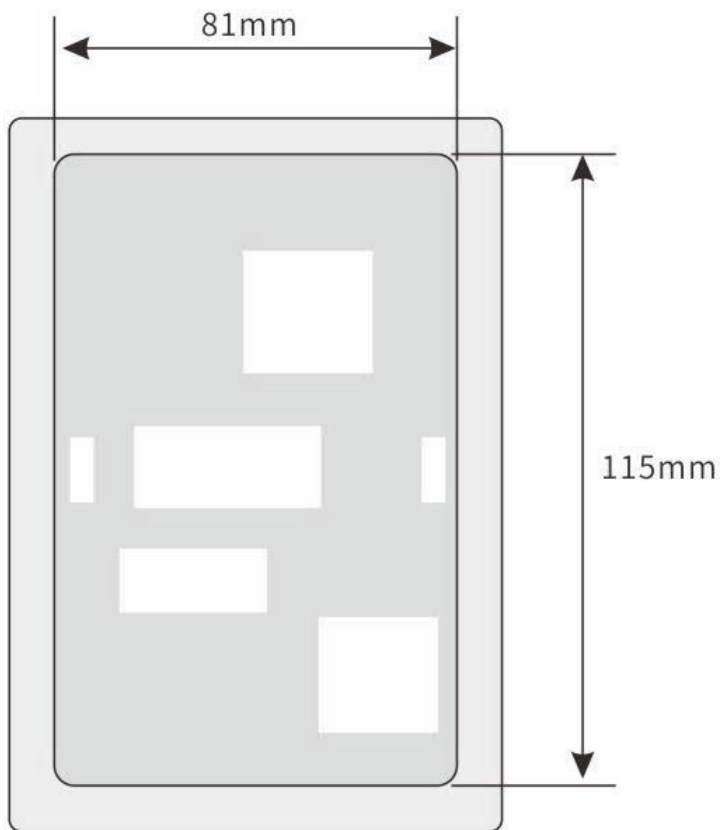
托盘开孔尺寸
