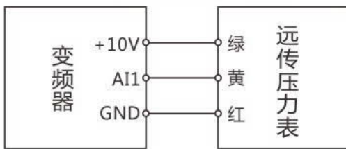
远传压力表接线图
