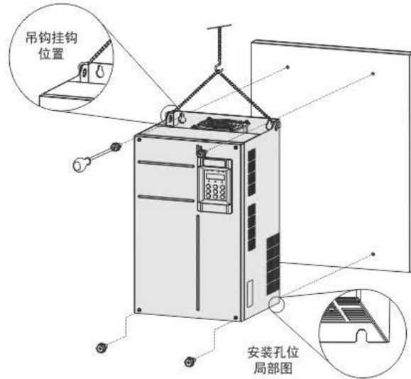
图 3-3 RDI67ST45G(B)~RDI67ST160G, RDI67S-2T22G(B)~RDI67S-2T55G机型壁挂式安装示意图
