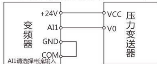
压力变送器接线图(4-20mA)
