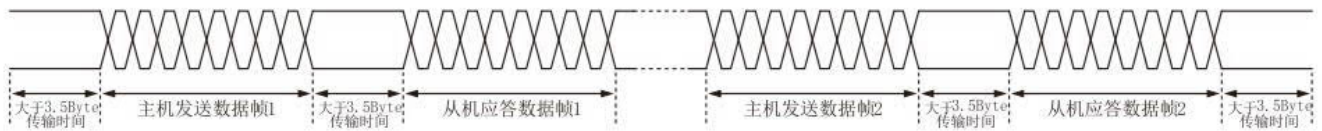
图 8-1 Modbus-RTU 数据传输示意图
