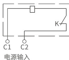
图1 AC 230V、400V、DC 24V接线图
