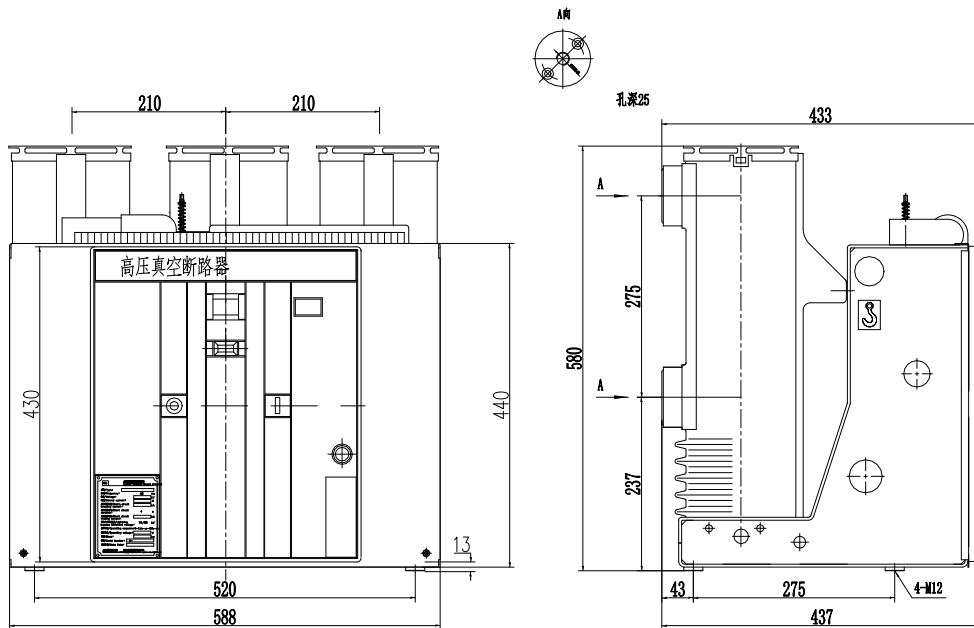
图3 固定式断路器外形尺寸图
