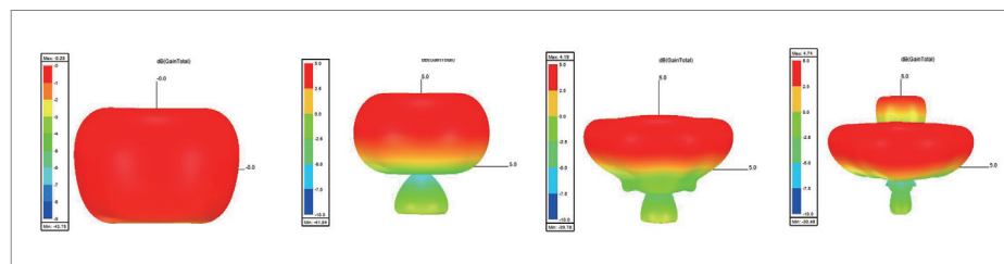
宽带全向天线 3D 方向图
