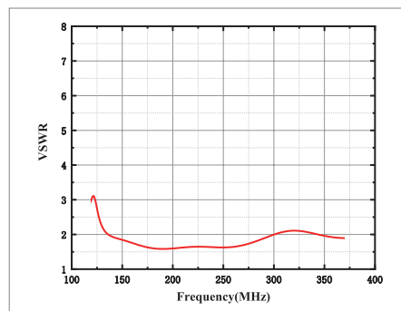
宽带全向天线驻波比
