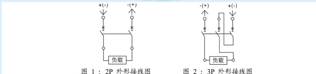
图 1：2P 外形接线图
